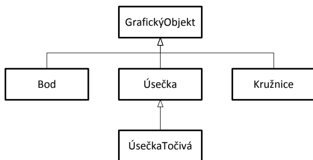
Obrázek 1.6: Dědická hierarchie tříd z příkladu o grafickém editoru
