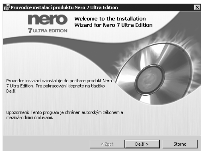
Obr. 1.4: Průvodce instalací
