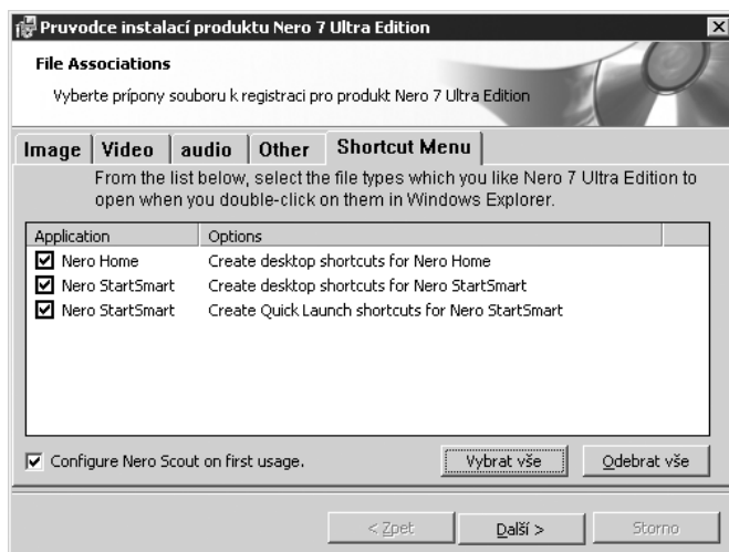
Obr. 1.10: Dokončení instalace
