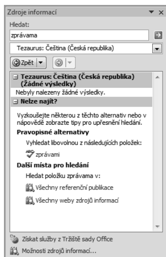
Obrázek 1.12: Pravopisné alternativy
