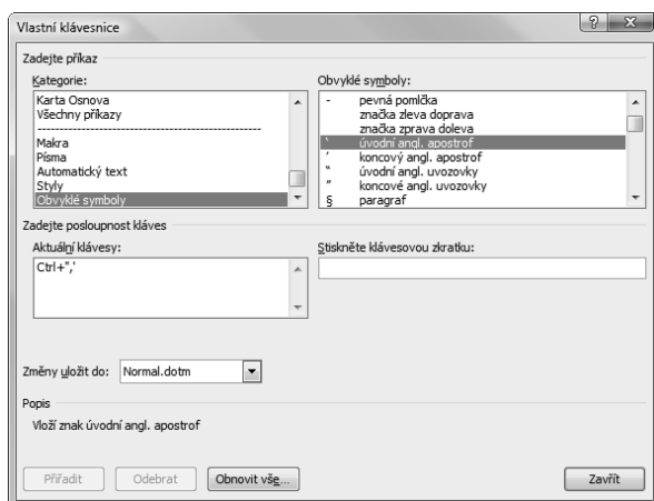
Obrázek 1.5: Obvyklé symboly
