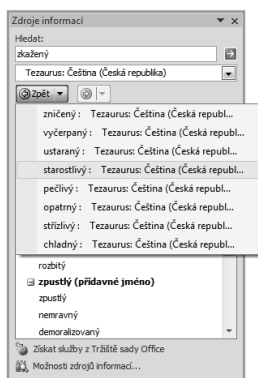
Obrázek 1.11: Možnosti tezauru
