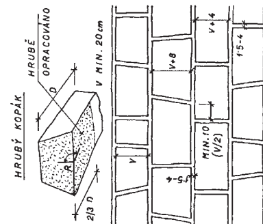
LÍC OBYČEJNÉHO HRUBÉHO ZDIVA ŘÁDKOVÉHO.
