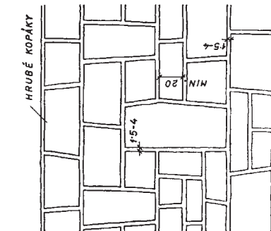
LÍC SVISLE PROVAZOVANÉHO HRUBÉHO ZDIVA ŘÁDKOVÉHO.
