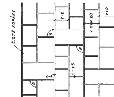
LÍC SVISLE PROVAZOVANÉHO ČISTÉHO ZDIVA ŘÁDKOVÉHO.
