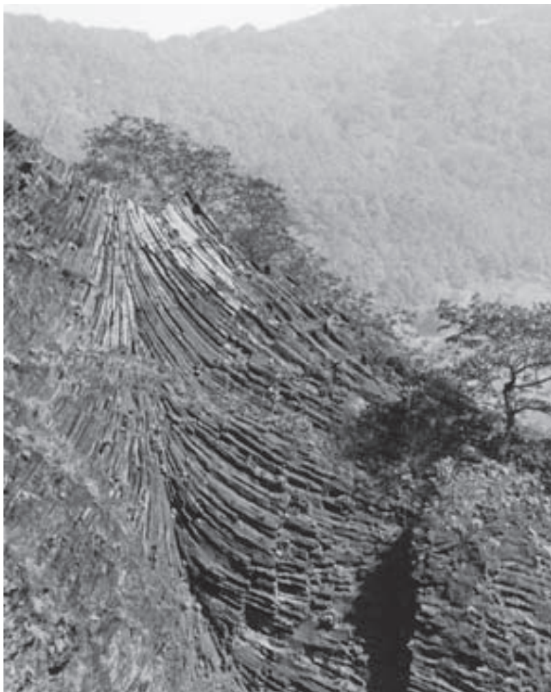
Sloupovitá odlučnost bazaltu neboli čediče (Vrkoč u Ústí nad Labem).
