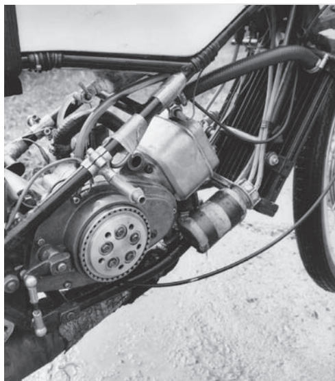
Oboustranný pohled na kapalinou chlazený motor jednoválce Ahra 50
