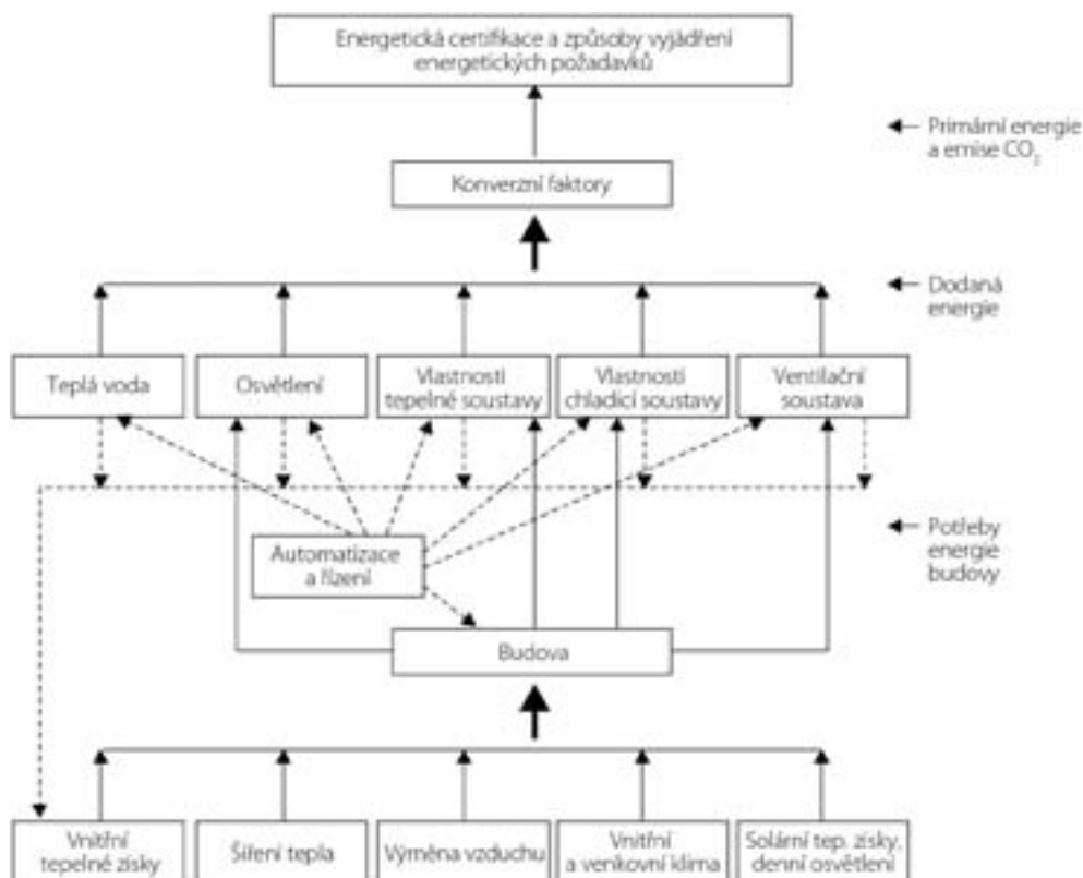
Obr. 2.3 Energetické toky a procesy [127]
