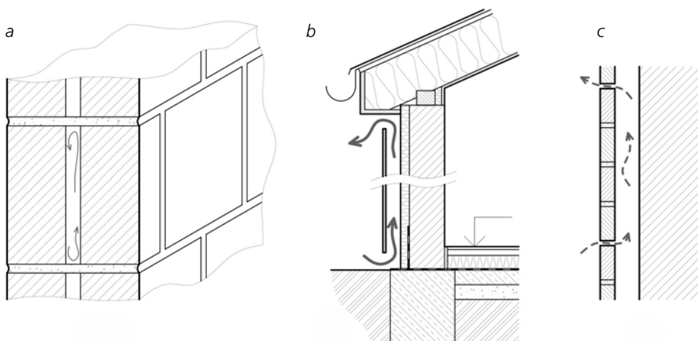
Obr. 1.4 Vzduchová vrstva: a) nevětraná; b) větraná (otevřená); c) slabě větraná
