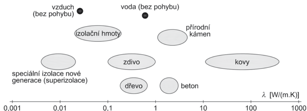
Obr. 1.2 Tepelná vodivost vybraných hmot (logaritmická stupnice)
