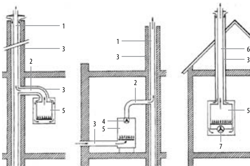
a) koncentrický přívod vzduchu komínem
