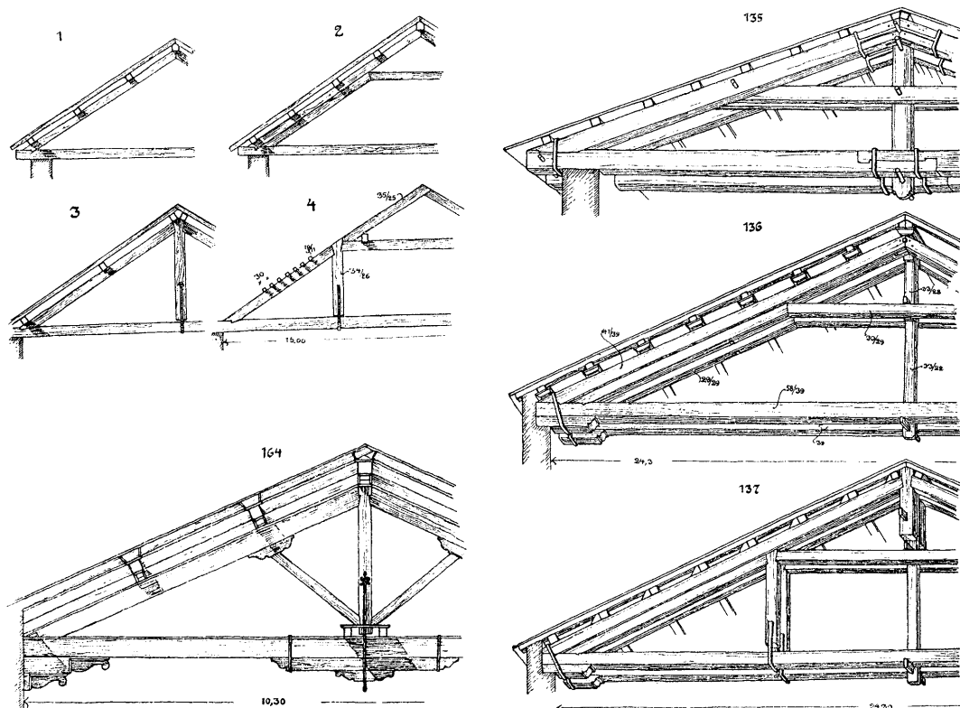
Typy vazníkových krovů [Ostendorf, 1908, viz str. 27]
