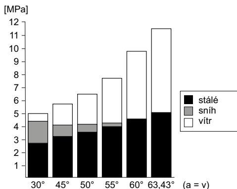
Obr. 2.4 Závislost namáhání krokví na sklonu střechy
