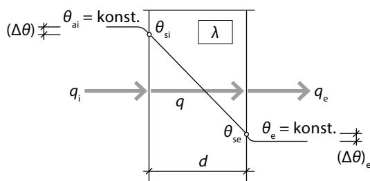
3 Schematické znázornění průběhu teplot jednovrstvou homogenní konstrukcí obvodového pláště s vlivem přestupu tepla na vnitřní a vnější straně konstrukce. Zdroj: CHMÚRNY, Ivan. Stavebná tepelná technika: Základy tepelnej ochrany budov. Bratislava: STU Bratislava. ISBN 978-80-227-4147-7, s. 59
