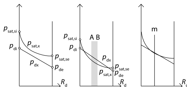
5 Schematické znázornění průběhu parciálních tlaků vodní páry jednovrstvou homogenní konstrukcí obvodového pláště bez kondenzace a s kondenzací. Zdroj: CHMÚRNY, Ivan. Stavebná tepelná technika: Základy tepelnej ochrany budov. Bratislava: STU Bratislava. ISBN 978-80-227-4147-7, s. 181
