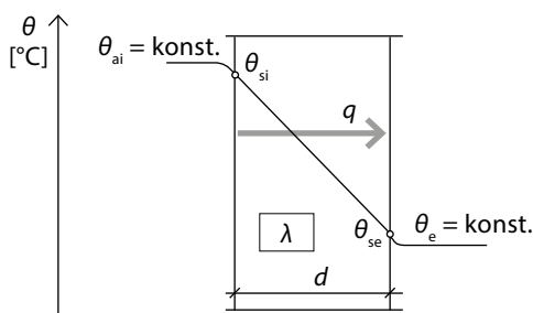
2 Schematické znázornění charakteristického průběhu teplot jednovrstvou homogenní konstrukcí obvodového pláště. Zdroj: CHMÚRNY, Ivan. Stavebná tepelná technika: Základy tepelnej ochrany budov. Bratislava: STU Bratislava. ISBN 978-80-227-4147-7, s. 52
