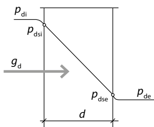
4 Schematické znázornění průběhu difuze vodních par jednovrstvou homogenní konstrukcí obvodového pláště s vlivem přestupu vodní páry na vnitřní a vnější straně konstrukce. Zdroj: CHMÚRNY, Ivan. Stavebná tepelná technika: Základy tepelnej ochrany budov. Bratislava: STU Bratislava. ISBN 978-80-227-4147-7, s. 180
