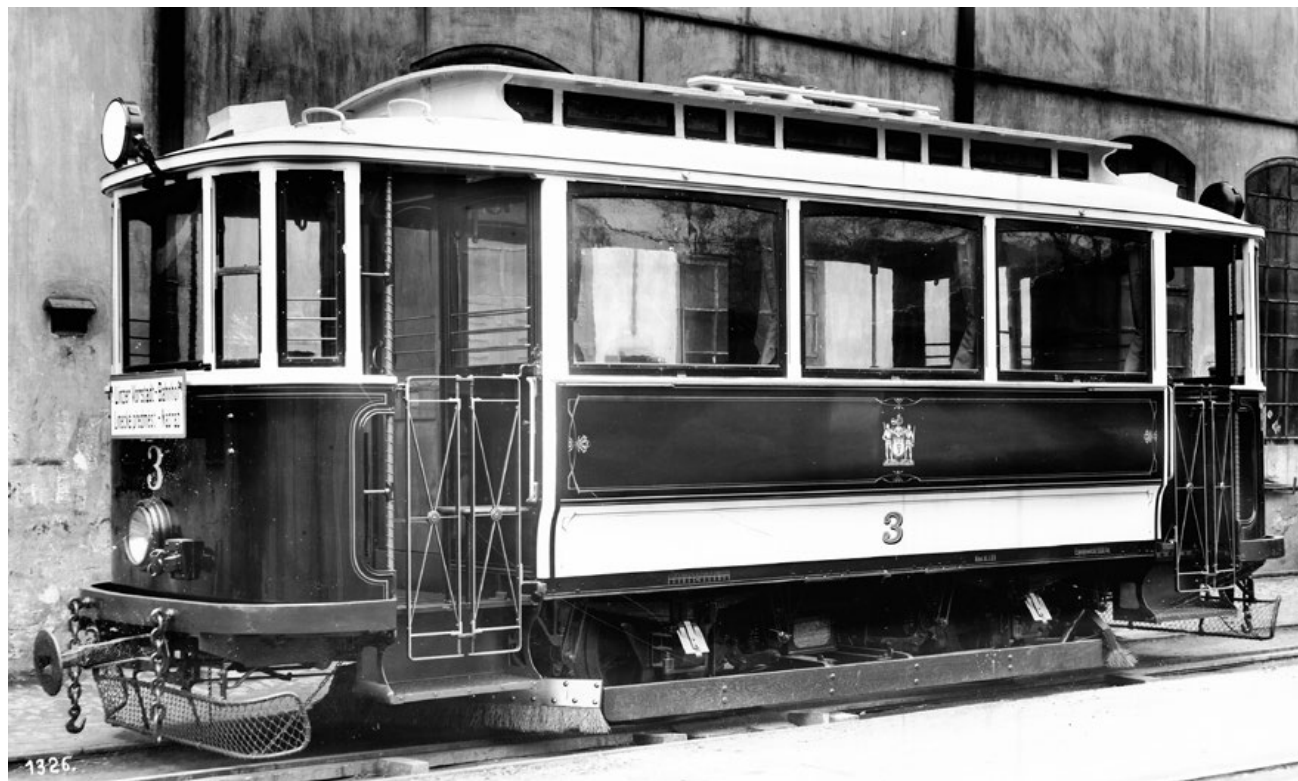
Tramvajový vůz číslo 3 ve stavu po vyrobení v roce 1909 v Ringhofferově strojárně
