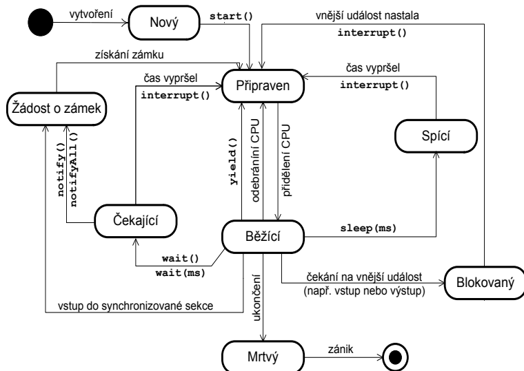
Obrázek 1.1 Diagram stavů podprocesu v Javě
