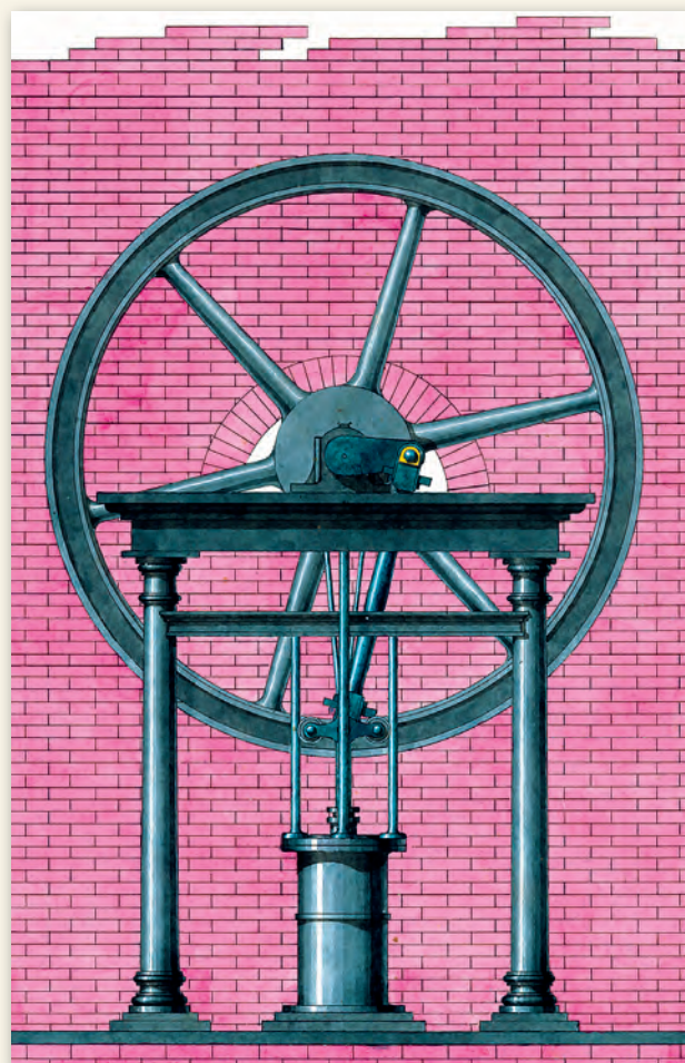
Stojatý parní stroj s invertním válcem mezi litinovými sloupky a s mohutným setrvačником (školní výkres strojnika Johanna Baleye, 28. 4. 1870)
