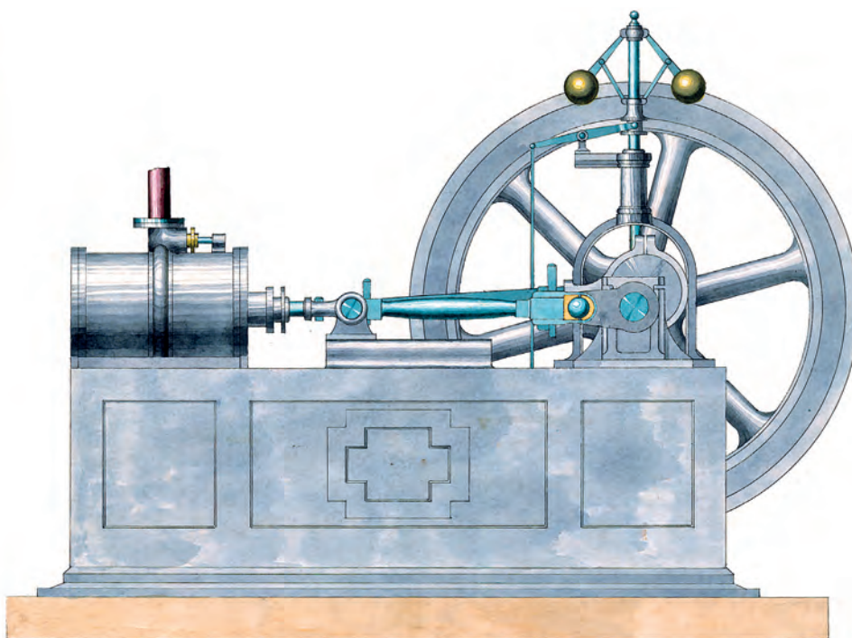
Ležatý parní stroj soustavy Duff s Wattovým odstře- divým regulátorem (školní výkres strojni- ka Johanna Baleye, 31. března 1870)
