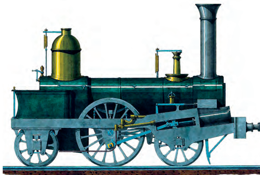
Jednosprežní parní lokomotiva pro dopravu osobních vlaků se skloněnými parními válci a plochými šoupátky. Na výkrese je patrné uspořádání náprav 1A1, vnější rám a vysoký parojem na kotli (školní výkres strojníka Johanna Baleye z období let 1866 – 1870)
