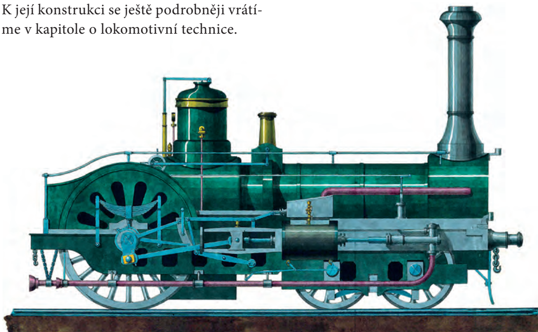
Jednosprežní parní lokomotiva soustavy Crampton pro dopravu rychlíků s kulisovým rozvodem soustavy Gooch a s uspořádáním náprav 2'A (školní výkres strojníka Johanna Baleye z období let 1866 – 1870)
