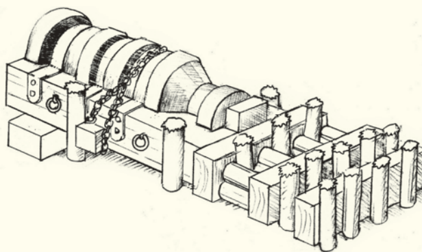
Zalafetovaná bombardra (podle P. Kubely)
