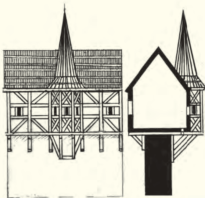
Krytý ochoz (15. století, podle Jaroslava Herouta)
