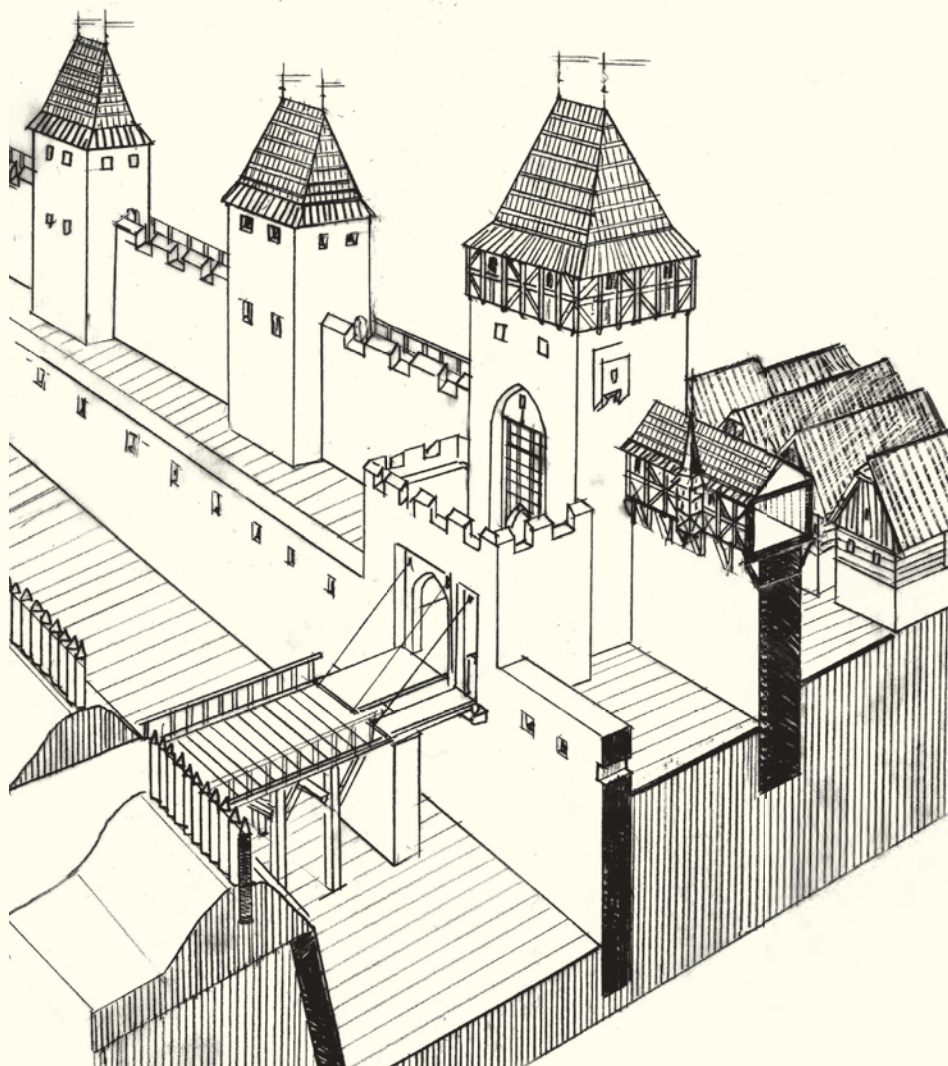
Brána (Tomáš Durdík, podle Jaroslava Herouta)
