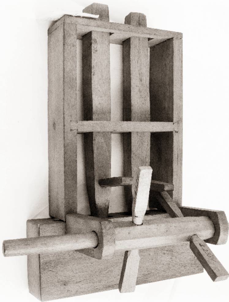
Model huculské tříselné stoupy, tzv. lubu. V rámu se pohybují dva svisle stojící bijany, které drtí kůru na tříslo. Mechanismus pohánějí za pomoci vodní síly lopatky na vodorovné hřídeli. Konec 19. století, ze sběrů Františka Řehoře na Podkarpatské Rusi.
