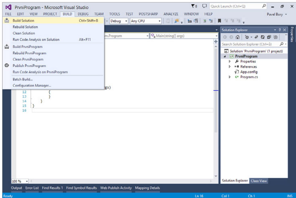
Obrázek 1.9 Build Solution
