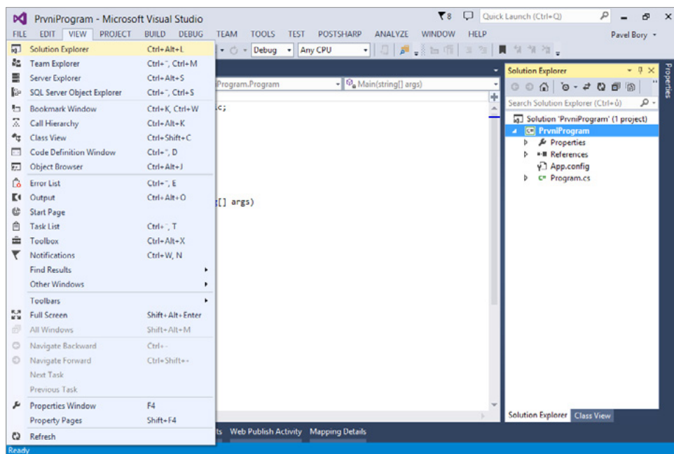
Obrázek 1.8 Solution Explorer
