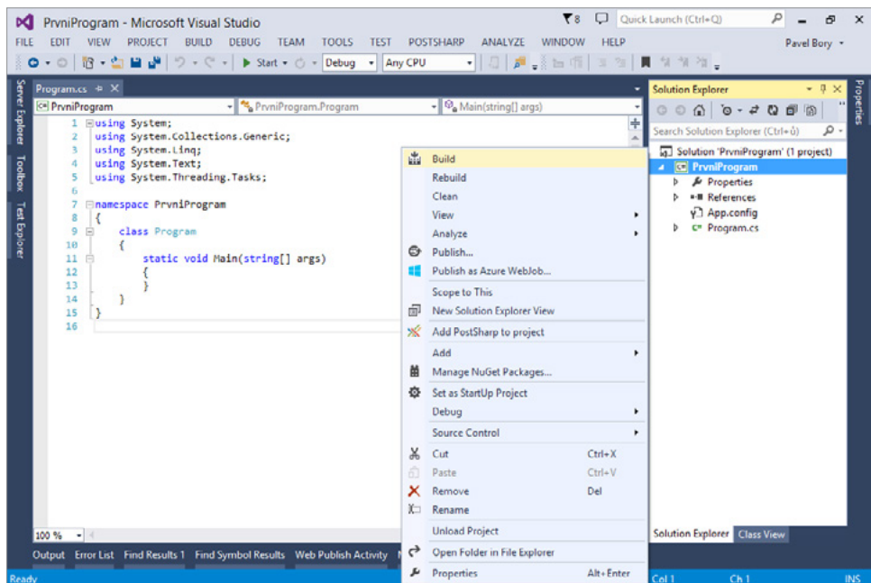
Obrázek 1.10 Build Project
