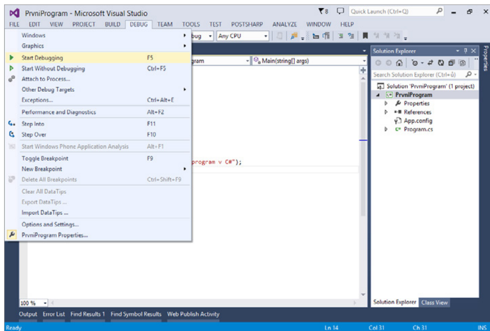
Obrázek 1.4 Spuštění programu
