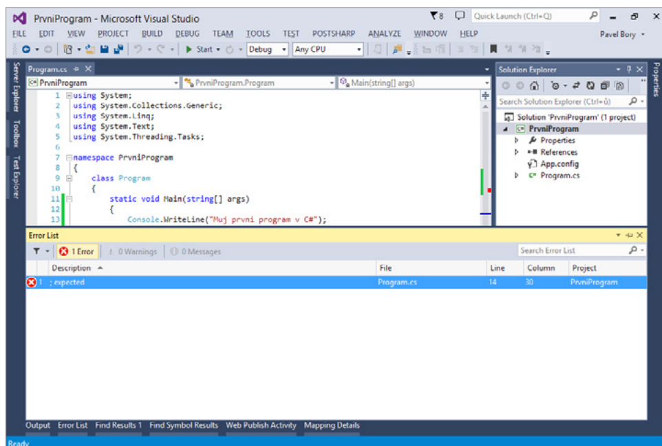
Obrázek 1.13 Error List
