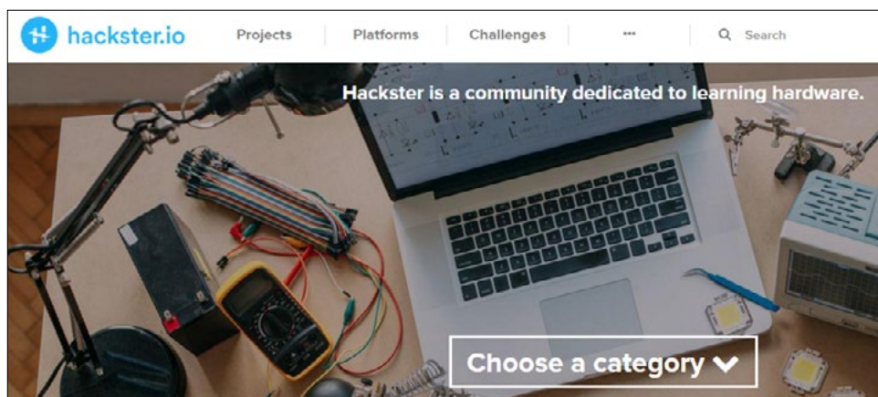
Obrázek 1.9: Portál Hackster
