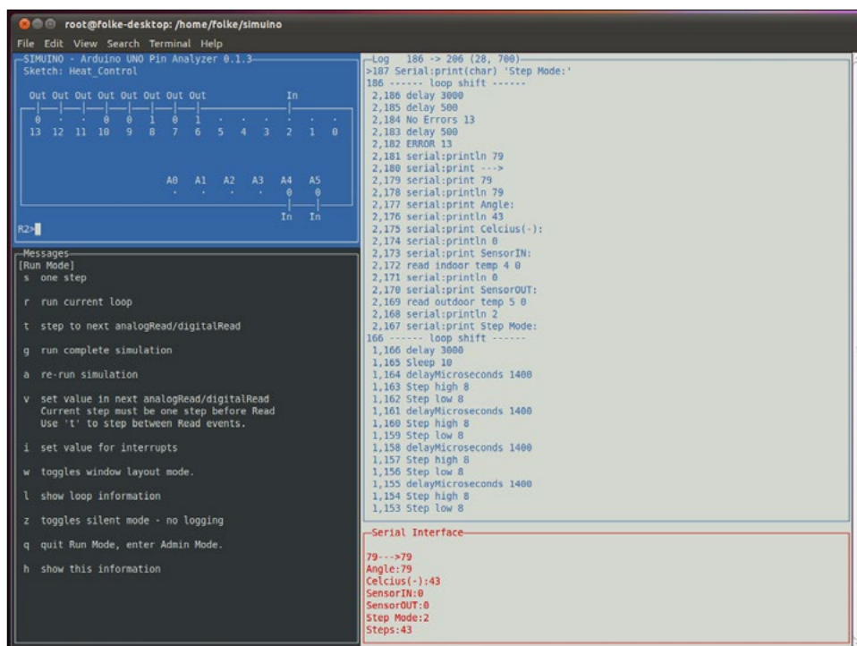
Obrázek 1.5: Simuino
