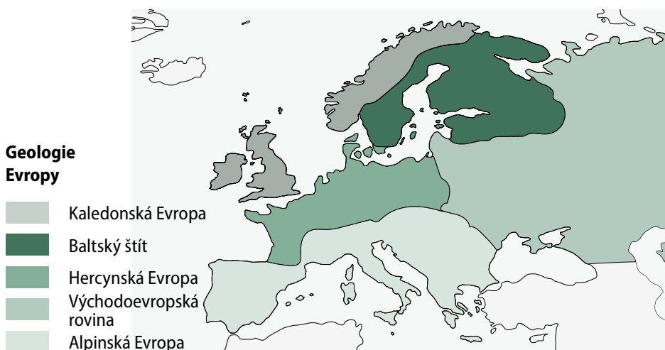
Geologie Evropy
