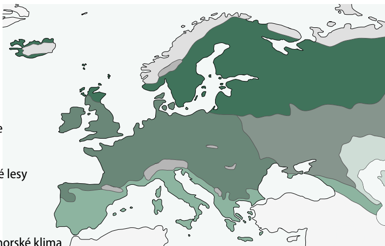
Biomy Evropy
