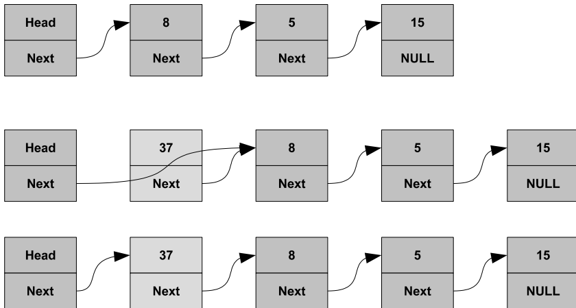
Obrázek 1.9: Jednosměrný spojový seznam
