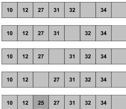
Obrázek 1.6: Přidávání doprostřed pole
