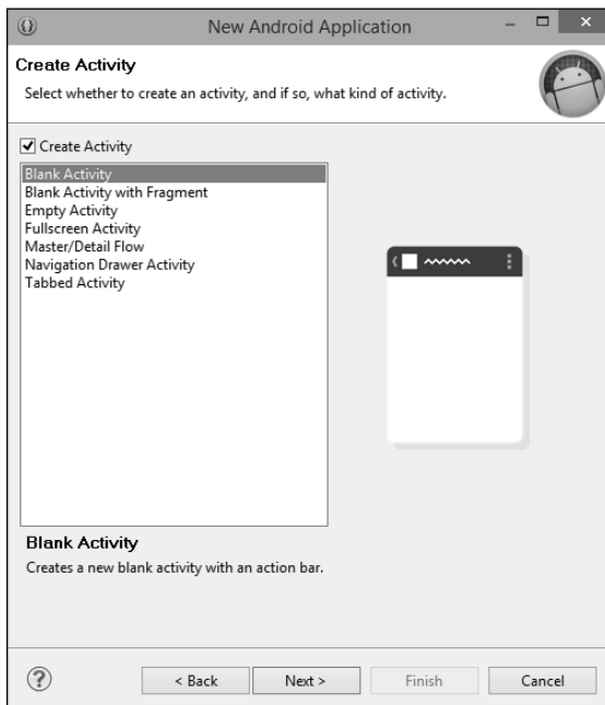
Obrázek 1.20: Vytvoření aktivity
