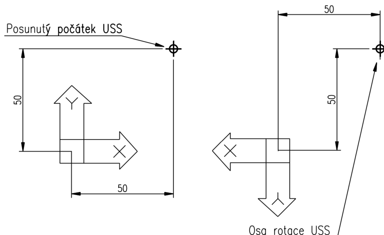
Obrázek č. 2.18: Rotace souřadného systému
