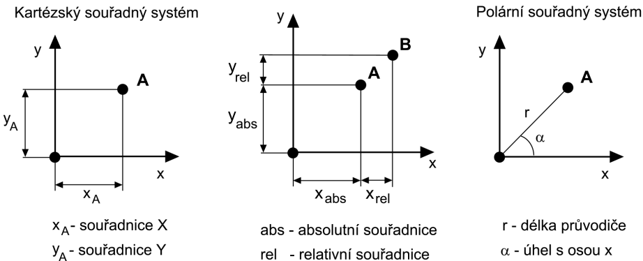
Obrázek č. 2.14: Druhy 2D souřadných systémů
