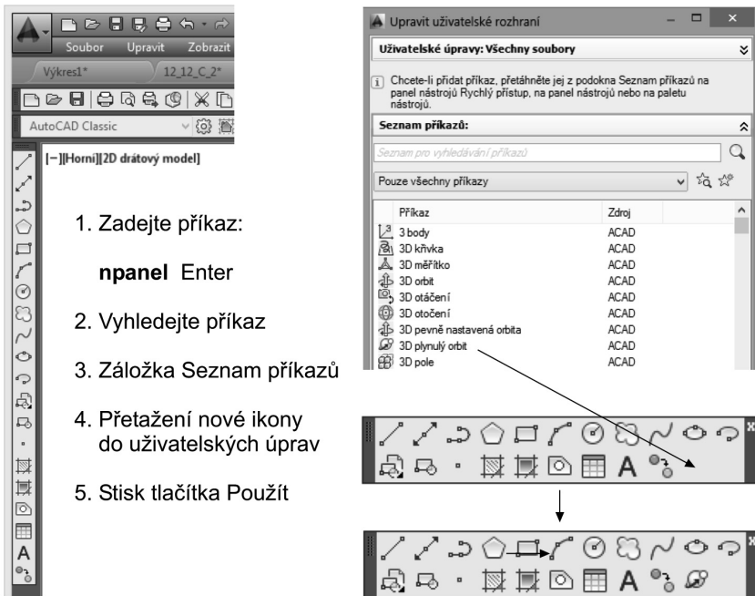
Obrázek č. 2.9: Modifikace panelu nástrojů přetažením ikony funkce
