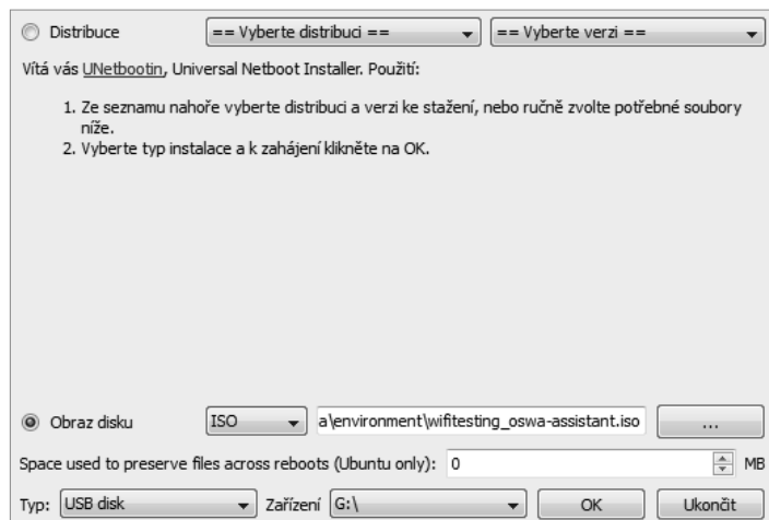
Obrázek 1.1 Unetbootin
