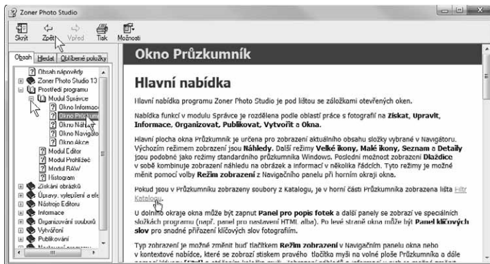
Obrázek 1.2: Okno nápovědy
